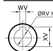
FIXO SAÍDA
