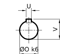
EIXO ENTRADA
