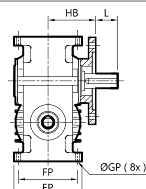
FIXO SAÍDA
