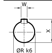
EIXO SAÍDA
