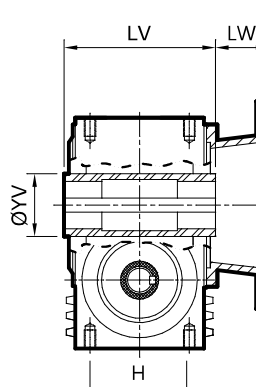
EIXO ENTRADA
