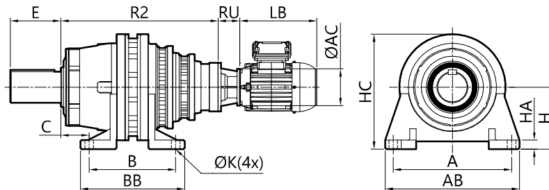
FIXAÇÃO PELA CARCAÇA MONTAGEM COM MOTOR - EIXO SAÍDA MACIÇO
