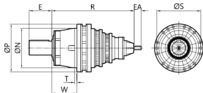
FIXAÇÃO PELA CARCAÇA MONTAGEM AP - EIXO OCO ESTRIADO
