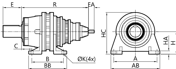
FIXAÇÃO PELA CARCAÇA MONTAGEM AP - EIXO SAÍDA MACIÇO
