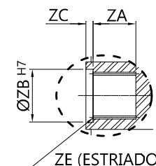
MONTAGEM COM EIXO OCO ESTRIADO
