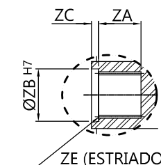
MONTAGEM COM EIXO OCO ESTRIADO
